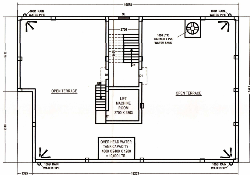
TERRACE PLAN SCALE- ( 1 : 100 )
